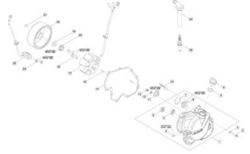
TAV.12 Gruppo accensione elettronica - Electronic ignition assy. - Groupe allumage électronique - Elektronischezündung gruppe - Grupo encendido electrónico
