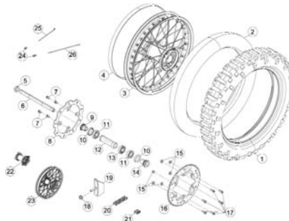
TAV.28 Ruota posteriore - Rear wheel - Roue AR. - Hinterrad - Rueda trasera
