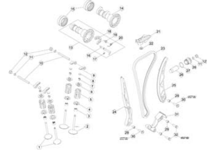
TAV.14 Valvole-Catena distribuzione - Valves-Timing chain - Soupapes-Chaine de distribution - Ventil-Steuerkette - Válvulas-Cadena de distribución
